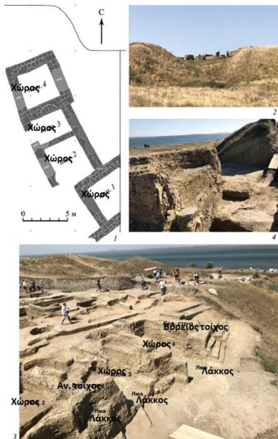
Εικ.82: τμήμα της αρχαϊκής οχύρωσης στην ΒΑ άκρη του λόφου της Ακρόπολης, Φαναγόρεια. 1: Σχεδιαστική αναπαράσταση οχύρωσης. 2: Άποψη οχύρωσης από τον βορρά. 3: Άποψη οχύρωσης από το νότο. 4: Τοίχος ανάμεσα στους χώρους 3-4. (Kuznetsov 2018β, εικ. 1. Επεξεργασία: Α. Μαστοράκου)
