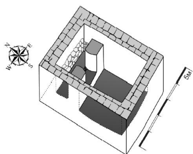
Εικ.80: Αξονομετρικό σχέδιο Ιερού 835. Β΄μισό 6ου αι. π.Χ.- Α΄μισό 5ου αι. π.Χ. Άνω Πόλη. Φαναγόρεια. (Kuznetsov 2019α, εικ.5)
