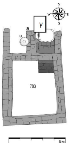
Εικ.76: Σχέδιο Ιερού 783. Γ΄ τετ. 6ου αι. π.Χ. Άνω Πόλη. Φαναγόρεια. α: βωμός, β: λεκάνη γ:λάκκος-βόθρος. (Kuznetsov 2019α, εικ.9. Επεξεργασία: Α. Μαστοράκου)
