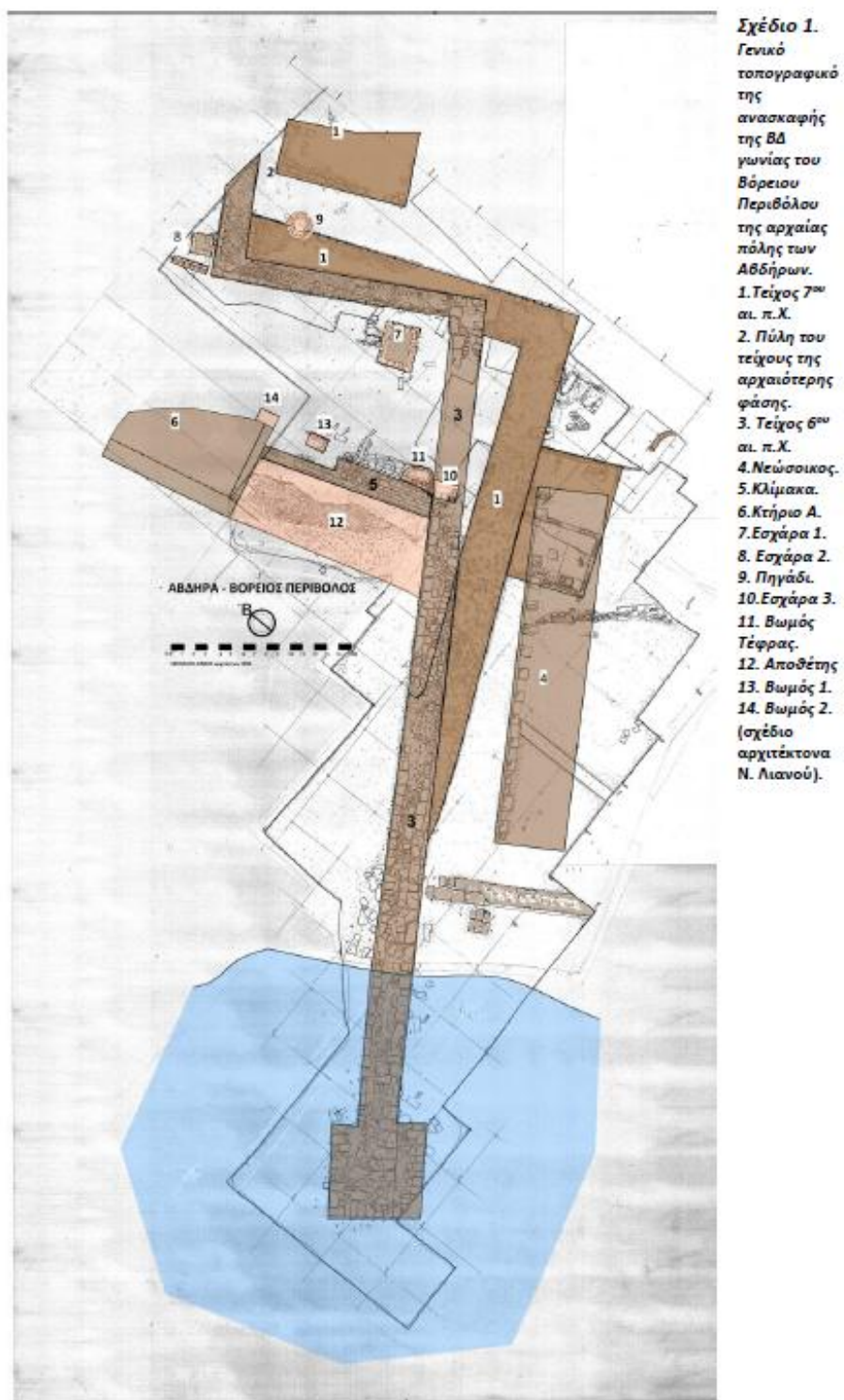
Εικ. 12: Γενικό τοπογραφικό της ανασκαφής της ΒΔ γωνίας του Βόρειου Περιβόλου. (Σαμίου-Λιανού 2019, σχ.1)
