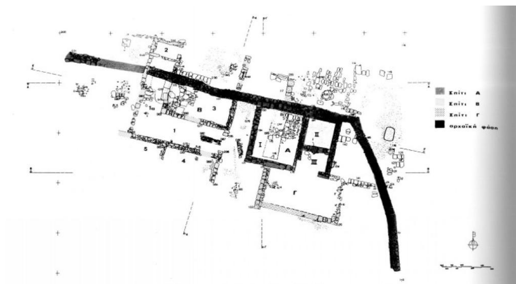
Εικ. 28: Ανασκαφική τομή, Βάλτα Ζαμπάκη. Άβδηρα. Κάτοψη. (Σκαρλατίδου 1992β, σχ.1)
