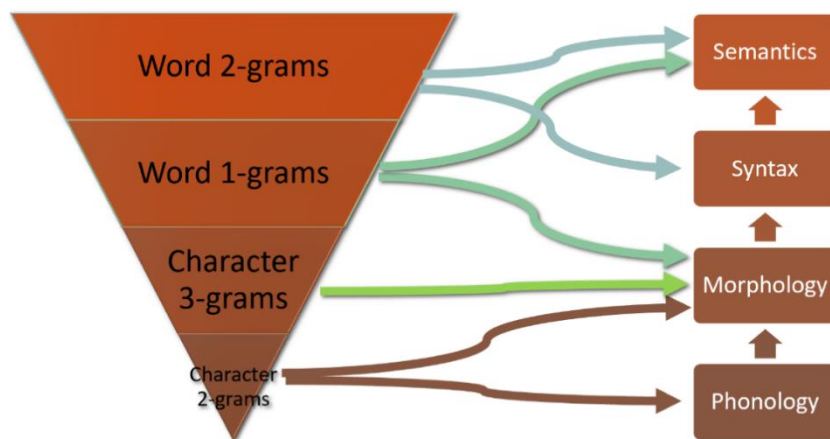
Εικόνα 2 AMNP: Μια ιεραρχική αναπαράσταση των χαρακτηριστικών ν-γραμμάτων και των αντίστοιχων γλωσσικών επιπέδων
