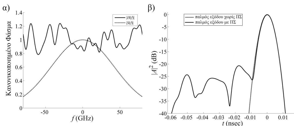
Εικόνα 4-9. α) Το φάσμα ενός Gaussian παλμού S(f) , το οποίο αντιστοιχεί σε ένα ρυθμό R_b=40\text{GHz} και το φάσμα εκπομπής που αντιστοιχεί στο φαινόμενο πολλαπλής σκέδασης, H(f) με συχνοτική απόσταση των ψευδοτυχαίων κορυφών στα 10\text{GHz} . β) Η κανονικοποιημένη ισχύς του παλμού εξόδου αγνοώντας το φαινόμενο της πολλαπλής σκέδασης (ΠΣ) και η κανονικοποιημένη ισχύς του παλμού λαμβάνοντας υπόψη το φαινόμενο ΠΣ, υπολογίζοντας το γινόμενο S(f)\cdot H(f) .
