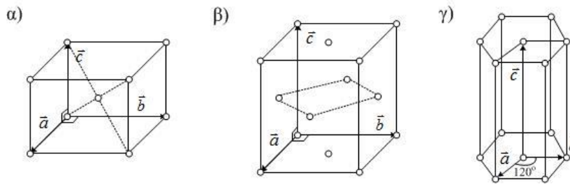
Εικόνα 2-4. α) Ορθορομβικό χωροκεντρωμένο (I) πλέγμα Bravais ( a \neq b \neq c ), β) Ορθορομβικό εδροκεντρωμένο (F) πλέγμα Bravais ( a \neq b \neq c ), γ) Εξαγωνικό (P) πλέγμα Bravais ( a = b \neq c , σε γωνία 120^\circ ).
