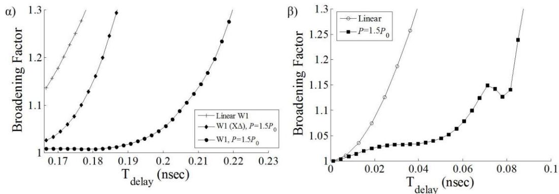
Εικόνα 4-16. Ο συντελεστής BF συναρτήσεσι της καθυστέρησης για (α) τους κυματοδηγούς W1 και W1 χαμηλής διασποράς (W1 ΧΔ) για R_b=100\text{Gb/s} (β) τον W1 ΧΔ διατηρώντας σταθερό n_g \cong 37 και επιλέγοντας μήκη μεταξύ 0 \leq L \leq \min(L_1, L_2) .
