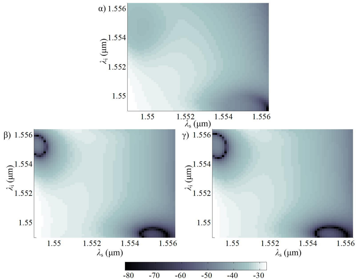
Εικόνα 5-5. Η απόδοσης μετατροπής \eta που παρουσιάζει ο ΚΦΚ που προτάθηκε από τους J. Li et al. [220], συναρτήσει των μηκών κύματος του σήματος και του ανεγειρόμενου κύματος, υπολογίζοντας α) αριθμητικά τις εξισώσεις (5.12)-(5.14) χρησιμοποιώντας μία υλοποίηση Runge-Kutta και υπολογίζοντας την αναλυτική έκφραση (5.36) με την ισχύ άντλησης να περιγράφεται β) από την υποενότητα 5.5.1 και γ) από την υποενότητα 5.5.2, αντίστοιχα.
