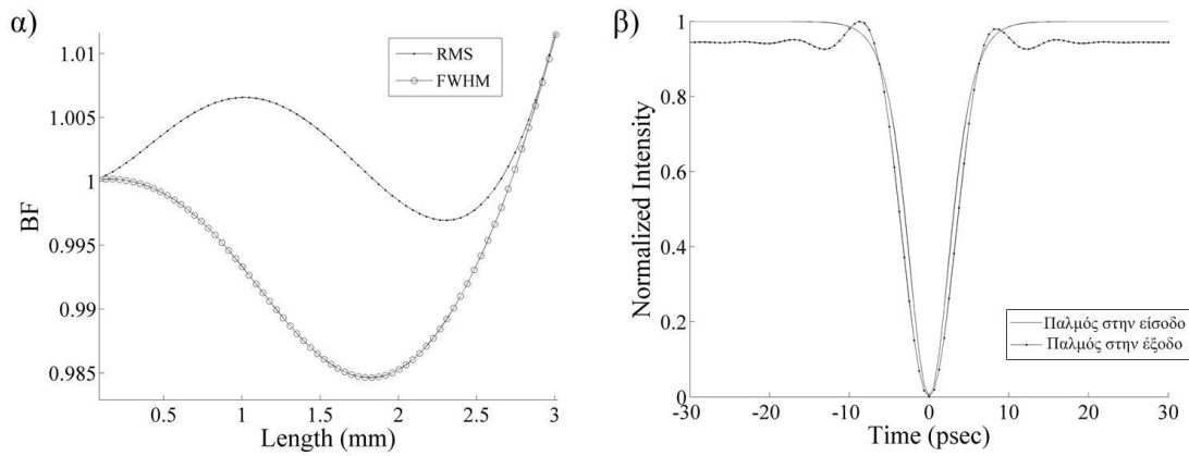
Εικόνα 4-15. (α) Συντελεστής BF και BF_{FWHM} συναρτήσεσι του μήκους διάδοσης, (β) ο αρχικός και ο τελικός παλμός για R_b=40\text{Gb/s} σε έναν W1 κυματοδηγό.
