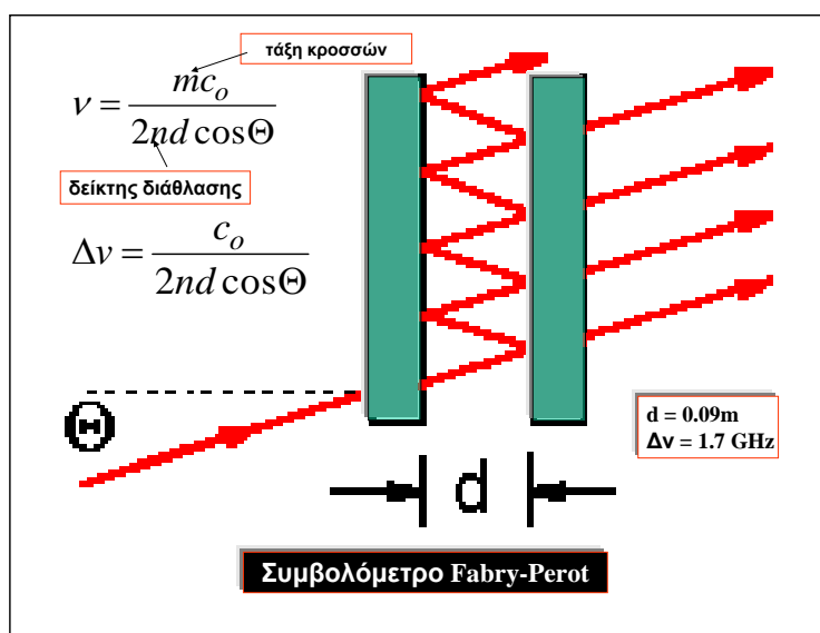
Εικόνα 9. Σχηματική περιγραφή λειτουργίας συμβολόμετρου Fabry-Perot. Στο Fabry-Perot σάρωσης η γωνία \Theta είναι 0^\circ και το εύρος του, d , μεταβάλλεται περιοδικά μέσω του πιεζοηλεκτρικού φαινομένου.
