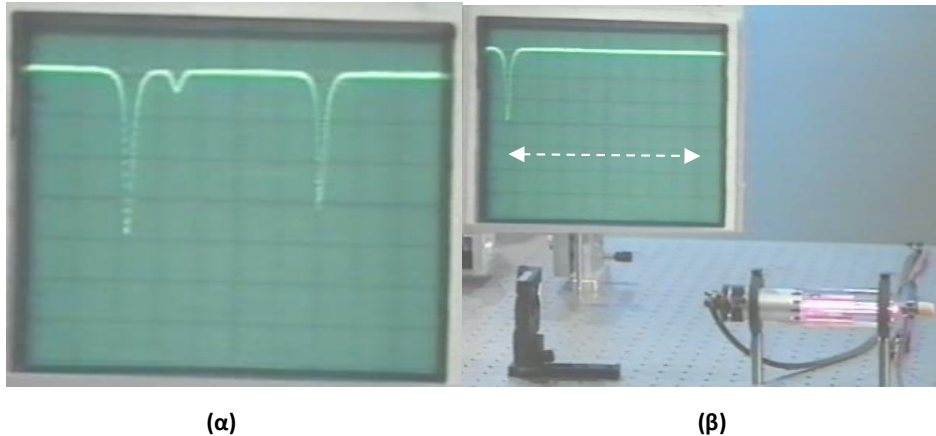
Εικόνα 16. (α) Φάσμα με δύο γραμμές δέσμης laser ( 1^{η} ς τάξης) από λυχνία με εσωτερικά κάτοπτρα, χωρίς παράθυρα σε γωνία Brewster. Το στοιχείο μικρής έντασης που φαίνεται ανάμεσα στις 2 γραμμές είναι μια από τις γραμμές αυτές ανώτερης τάξης (β) Με περιστροφή του πολωτή απομένει μία συχνότητα που μετατοπίζεται κατά μήκος της οθόνης (κατά μήκος της διακεκομμένης γραμμής), όταν ψύχεται η λυχνία με εκτόξευση ψυχρού αέρα επάνω της.
