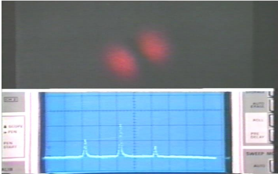
Εικόνα 31. Εάν το λεπτό σύρμα που βρίσκεται στο κέντρο της δέσμης περιστραφεί, τότε πάνω σε πέτασμα θα φανεί η το TEM_{01} να περιστρέφεται ανάλογα.
