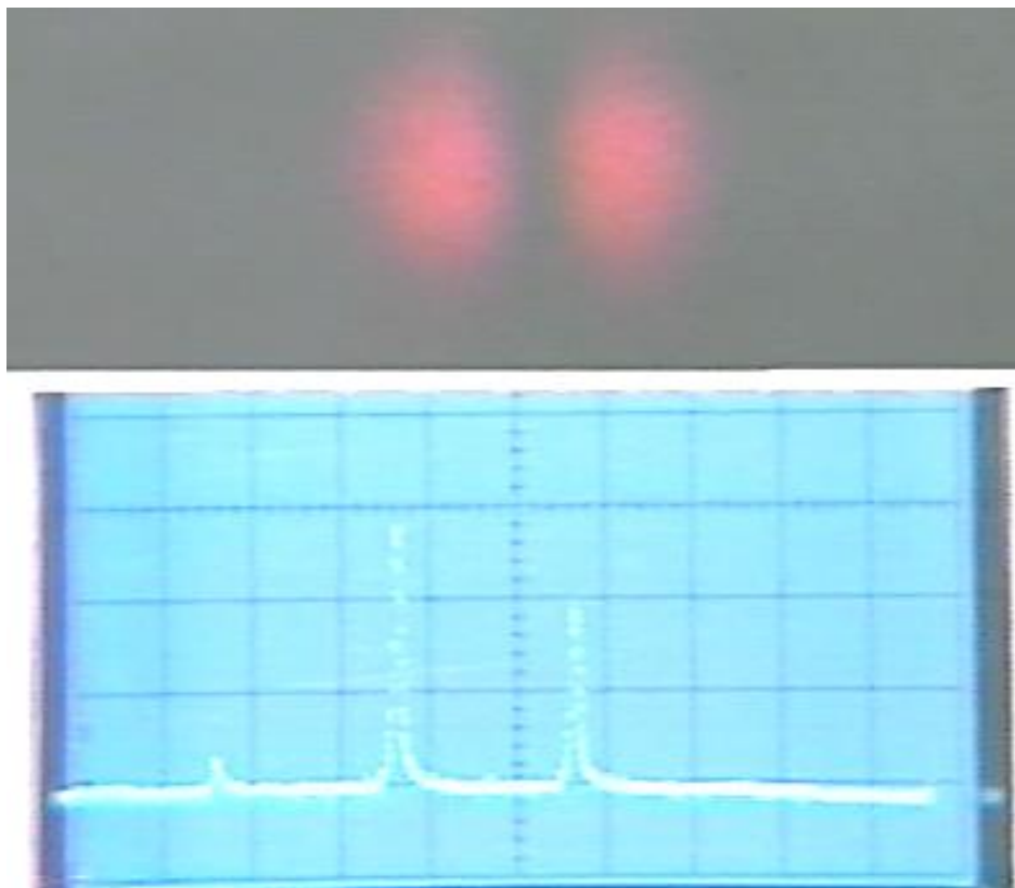
Εικόνα 29. Ο TEM 01 σε οθόνη (επάνω) που απομονώθηκε αφού τοποθετήθηκε ένα νήμα 50 μm στο κέντρο της δέσμης laser. Κάτω: Το φάσμα της σε παλμογράφο μέσα από συμβολόμετρο Fabry-Perot.
