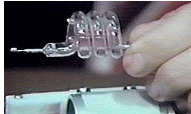
Εικόνα 4. Αριστερά: Ο Theodore H. Maiman επιδεικνύει τον ελικοειδή σωλήνα εκκένωσης για την άντληση του Ruby laser και την αλουμινένια θήκη του. Δεξιά: ο ελικοειδής σωλήνας εκλάμπσεων που χρησιμοποιείται για άντληση και επιτευξη αναστροφής πληθυσμού.
