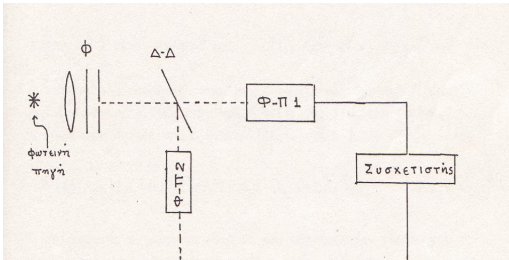
Εικόνα 40. Σχηματική διάταξη του πειράματος Hanbury-Brown & Twiss για τον προσδιορισμό της συνάρτησης συσχέτισης 2 ου βαθμού, G^{(2)} .
