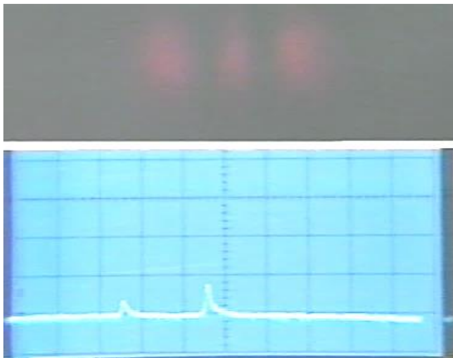
Εικόνα 30. Ο TEM02 που απομονώθηκε αφού τοποθετήθηκε ένα νήμα διαμέτρου 50 \mu\text{m} σε θέση όπου το πεδίο του είναι μηδέν (σκοτεινές περιοχές), και όπου το πεδίο των TEM01 και TEM00 είναι διάφορο του μηδενός.
