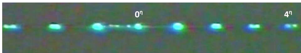
Εικόνα 19. Ανάλυση του φάσματος του laser ιόντων Αργού, Ar^+ με οπτικό φράγμα. Προσδιορίζεται στην εικόνα η περίθλαση μηδενικής και 4^{η} τάξης στην οποία οι γραμμές (στο μπλε, ανοιχτό μπλε και πράσινο) αρχίζουν να ξεχωρίζουν.
