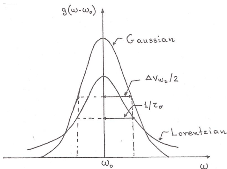
Εικόνα 23. Σύγκριση μεταξύ μιάς Λορεντζιανής και μιάς Γκαουσιανής μορφής φασματικής γραμμής. Έχουν σχεδιασθεί έτσι ώστε να έχουν το ίδιο εύρος στο μισό τους ύψος.
