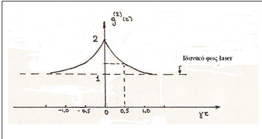
Εικόνα 37. Κανονικοποιημένη συνάρτηση συσχέτισης δευτέρου βαθμού χαώδους φωτεινής πηγής Λορεντζιανής φασματικής κατανομής, συγκρινόμενο με φως laser μίας συχνότητας και μίας μόνο TEM_{nlm} .
