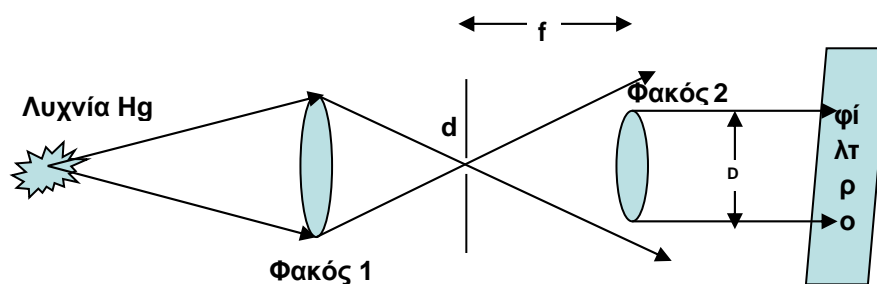
Εικόνα 1. Οπτικό τέχνασμα για να αποκτήσει ακτινοβολία συμβατικής φωτεινής πηγής (από λυχνία ατμών υδραργύρου) τις ιδιότητες της δέσμης laser.
