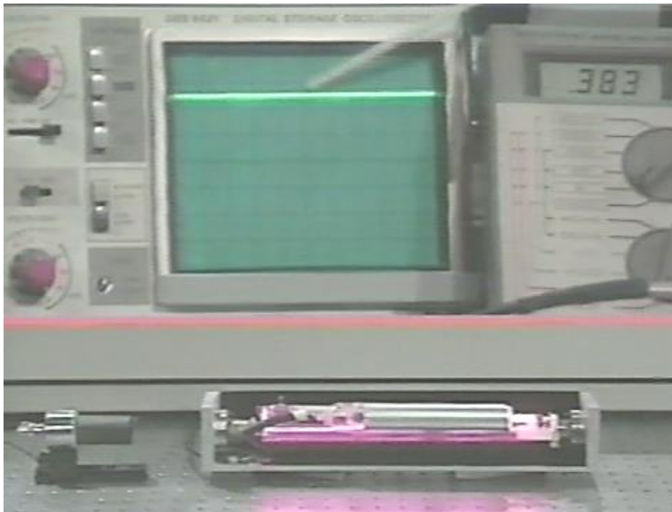
Εικόνα 18. Όταν ανάβει η λυχνία laser HeNe (B) εκπέμπεται η αυθόρμητη ακτινοβολία (ροζ απόχρωσης), ενώ το υλικό του υπό αναστροφή πληθυσμού ενισχύει τη δέσμη laser (A) από 364 mV στα 383 mV.
