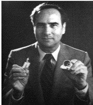
Εικόνα 4. Αριστερά: Ο Theodore H. Maiman επιδεικνύει τον ελικοειδή σωλήνα εκκένωσης για την άντληση του Ruby laser και την αλουμινένια θήκη του. Δεξιά: ο ελικοειδής σωλήνας εκλάμπσεων που χρησιμοποιείται για άντληση και επιτευξη αναστροφής πληθυσμού.
