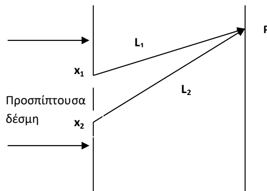
Εικόνα 38. Σχηματικό διάγραμμα συμβολόμετρου του Young
