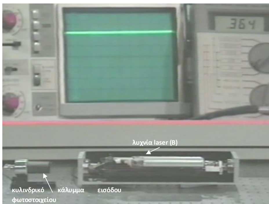
Εικόνα 17. Πάνω: Ο παλμογράφος δείχνει 364mV, ένδειξη που καταγράφει την ένταση της δέσμης laser (A) πριν να ενισχυθεί από το ενεργό υλικό της λυχνίας (B) που εμφανίζεται στην κάτω εικόνα.
