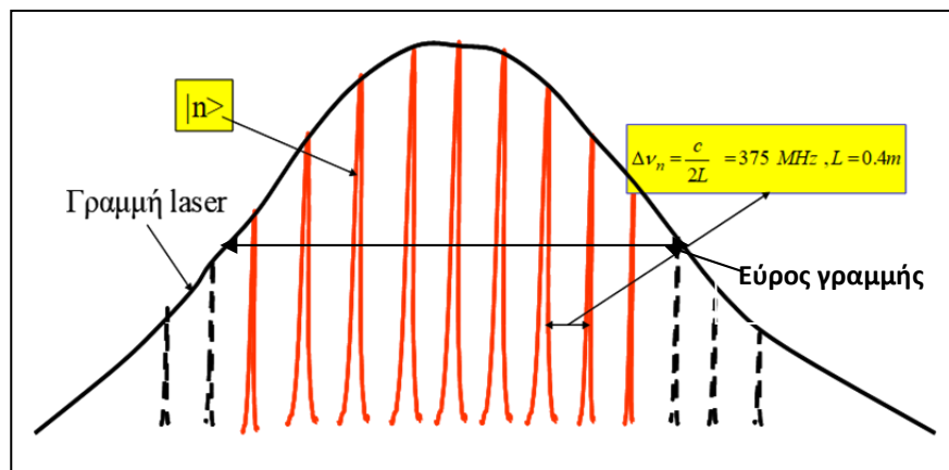
Σχήμα 10. Φάσμα διαμήκων συχνοτήτων της γραμμής laser. Η απόσταση μεταξύ τους είναι c/2L .
