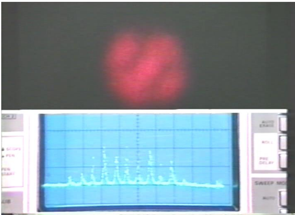
Εικόνα 28. Οι TEM_{lm} ανώτερης τάξης σε υπέρθεση έτσι όπως εμφανίζονται σε πέτασμα (επάνω) και στην οθόνη παλμογράφου (κάτω) αφού αναλυθούν από ένα συμβολόμετρο Fabry-Perot
