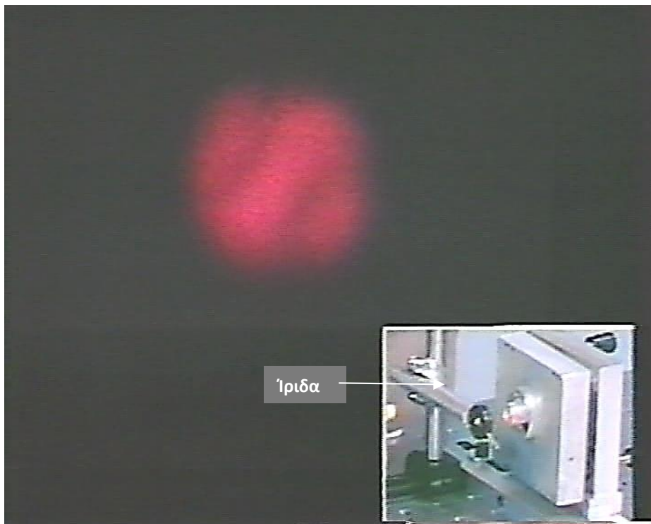
Εικόνα 25. Υπέρθυση πολλών εγκάρσιων τρόπων ταλάντωσης TEM_{lm} (όπως φαίνονται πάνω σε πέτασμα) μετά από μεγέθυνση με βοήθεια αποκλίνοντος φακού. Η ένθετη εικόνα δείχνει το κάτοπτρο της κοιλότητας και μία ίριδα τοποθετημένη μπροστά του για να αποκόψει τα ανώτερα TEM_{lm} .
