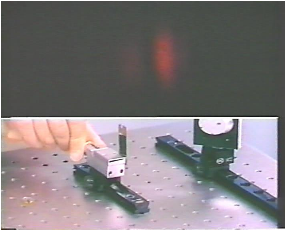
Εικόνα 32 Η λεπίδα ξυραφιού, τοποθετημένη έξω από την κοιλότητα συντονισμού, αποκόπτει μέρος του ενός λοβού της TEM_{01} ενώ ο άλλος λοβός δεν καταστρέφεται.
