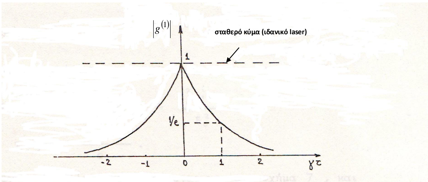
Εικόνα 36. Συμφωνία πρώτου βαθμού χαώδους φωτεινής πηγής με Lorentzian φασματική κατανομή. Το laser απεικονίζεται προσεγγιστικά σαν ένα σταθερό κύμα.
