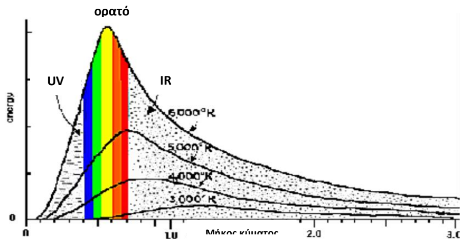
Σχήμα 2. Ένταση ακτινοβολίας μέλανος σώματος συναρτήσει του μήκους κύματος για διάφορες θερμοκρασίες. Το μέγιστο της έντασης ακολουθεί το νόμο του Wien, ανάλογο της τετάρτης δύναμης του T και για T=6000\text{K} βρίσκεται στη περιοχή του ορατού.
