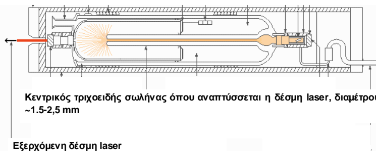
Εικόνα 24. Σχηματικό διάγραμμα της λυχνίας laser HeNe της εταιρείας Melles Griot
