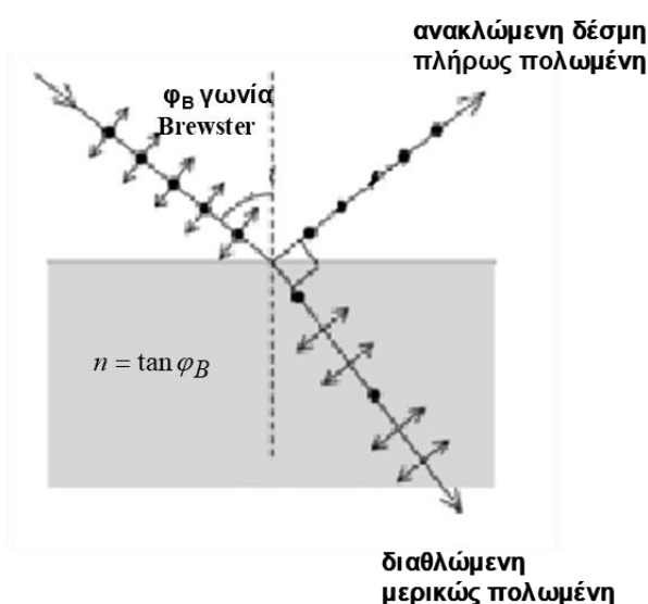
Εικόνα 13. Πόλωση ακτινοβολίας με ανάκλαση σε γωνία Brewster, ο σχετικός δείκτης διάθλασης είναι n .
