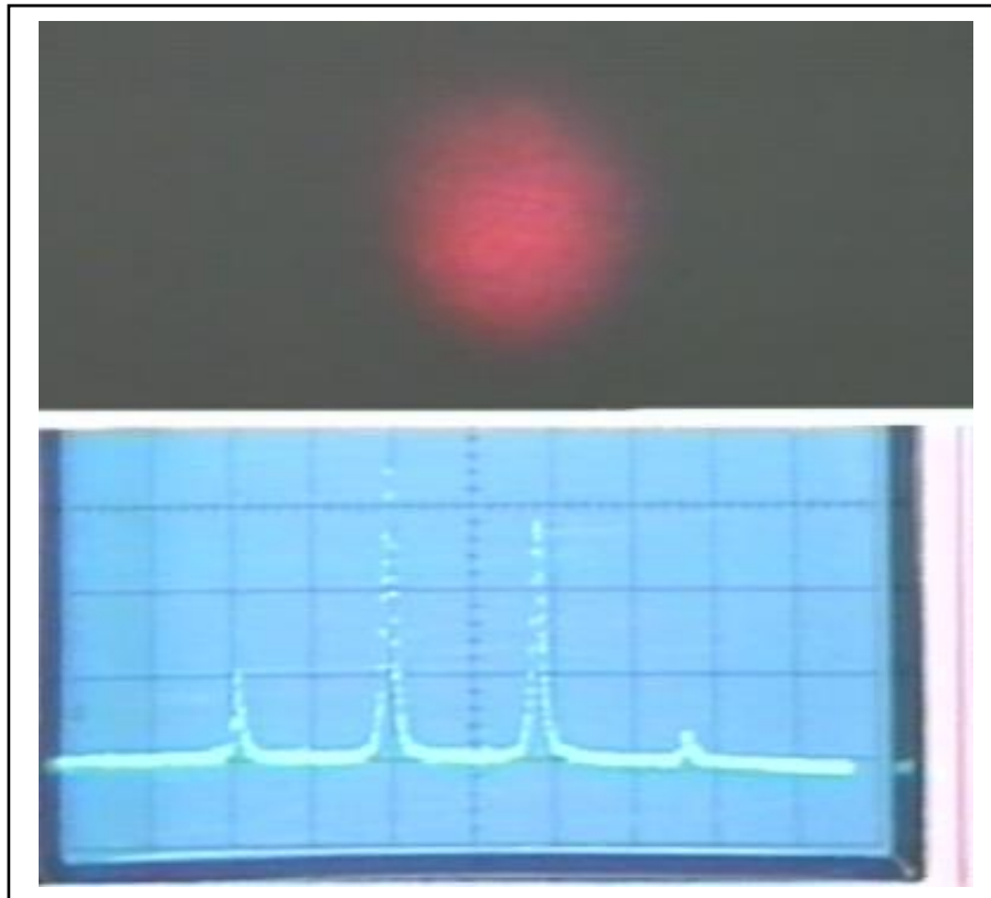
Εικόνα 27. Επάνω: Το αποτύπωμα της TEM_{00} επάνω σε πέτασμα. Κάτω: Οι τέσσερις διαμήκεις συχνότητες του όπως αναλύονται με συμβολόμετρο Fabry-Perot και εμφανίζονται σε οθόνη παλμογράφου.
