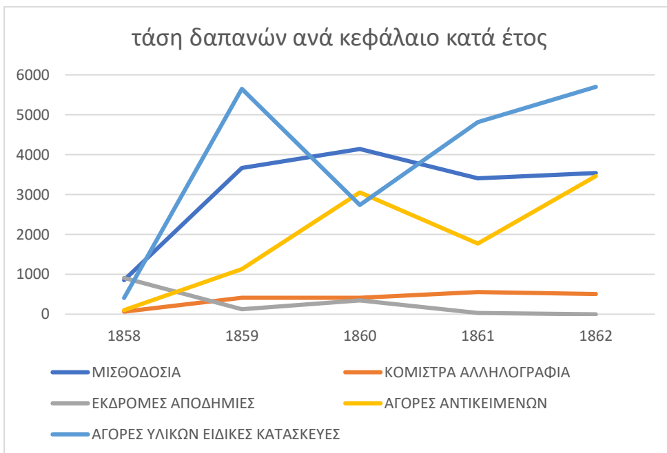
Εικόνα 55: Διάγραμμα τάσεων δαπανών ανά κεφάλαιο σε κάθε έτος
