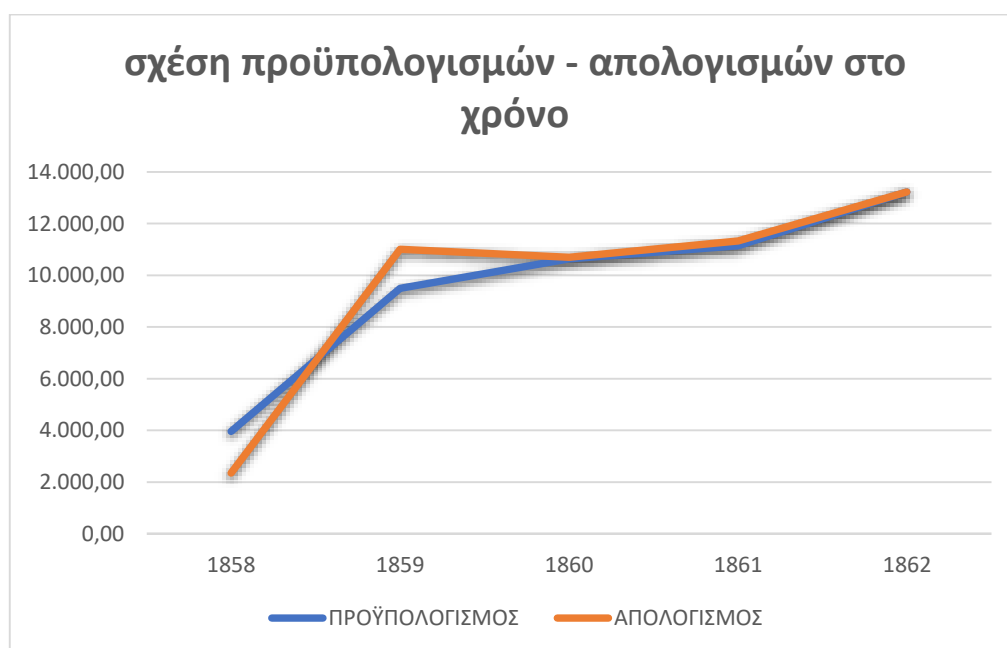
Εικόνα 53: Γράφημα απεικόνισης των τάσεων του προϋπολογισμού και του απολογισμού.
