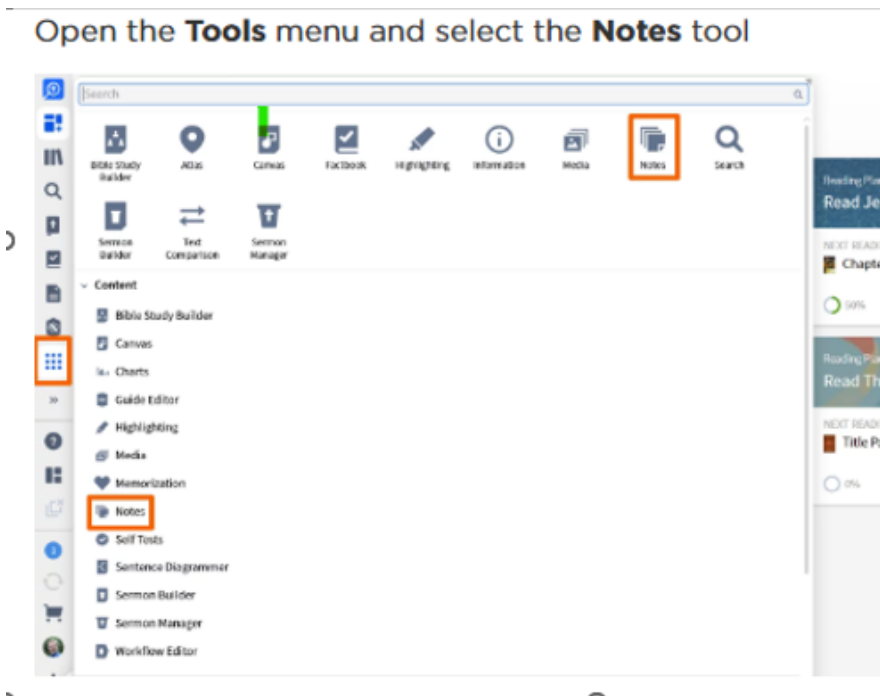
Εικόνα 65: Notes-Logos
