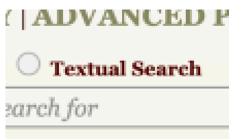
Εικόνα 14: Textual Search-TLG.
