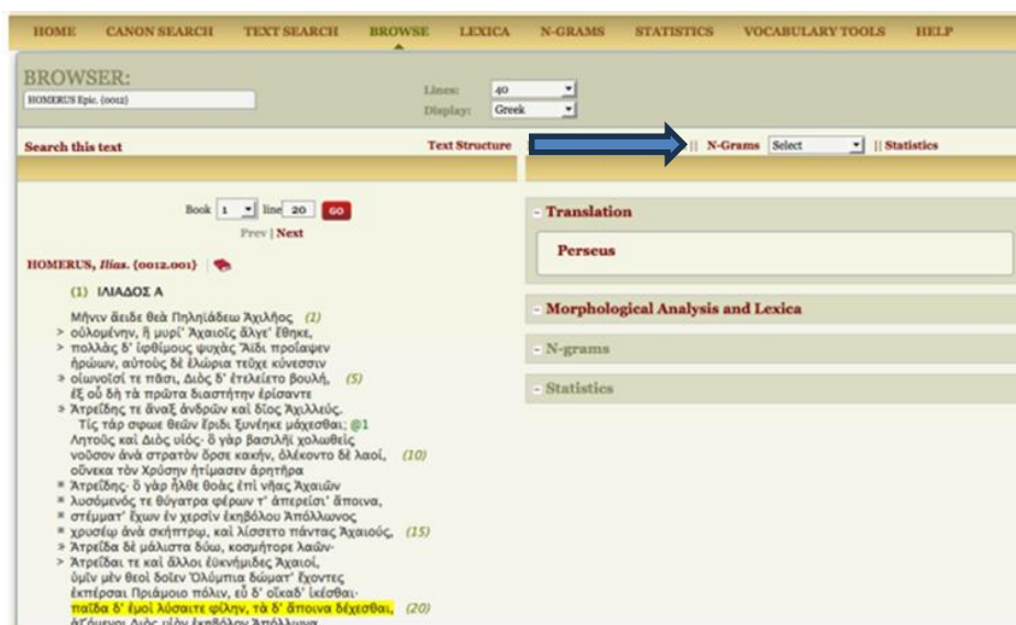
Εικόνα 21: Λειτουργία n-grams-TLG.
