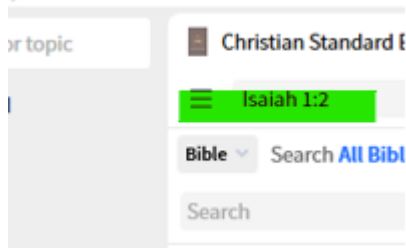
Εικόνα 67: Command Box-Logos.
