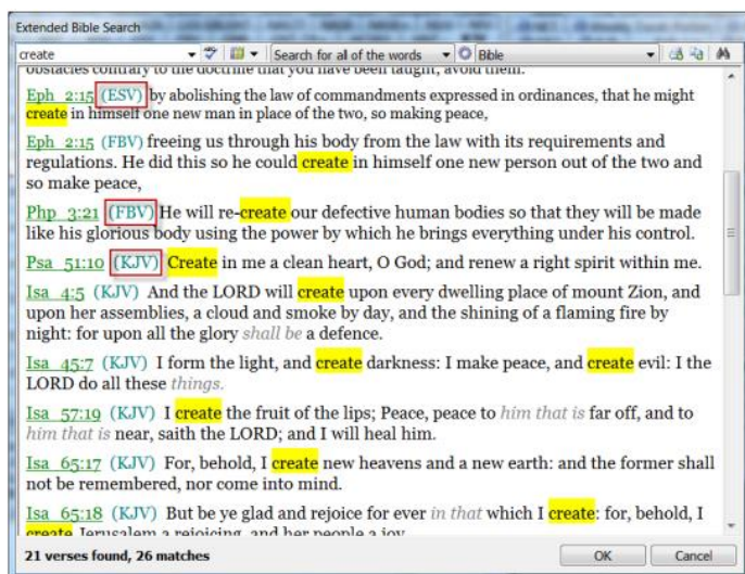
Εικόνα 48: Extended Search-e-Sword.
