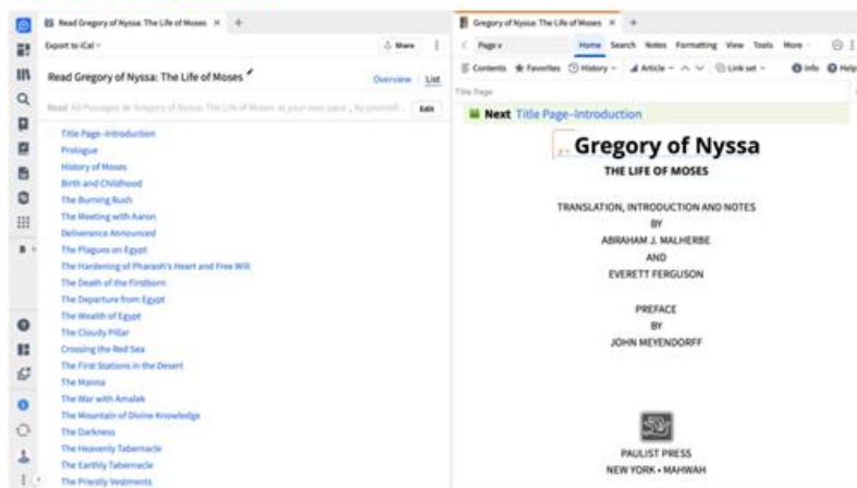
Εικόνα 62: Σχέδια μελέτης-Logos.
