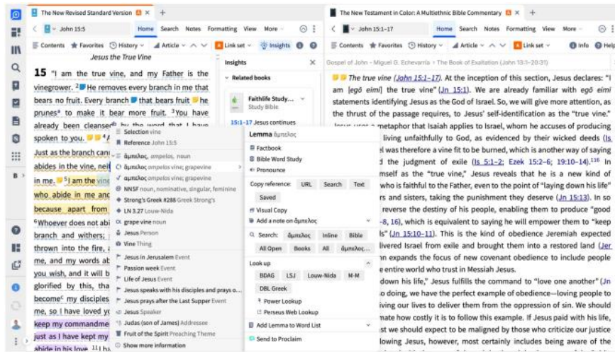
Εικόνα 59: Context menu-Logos.
