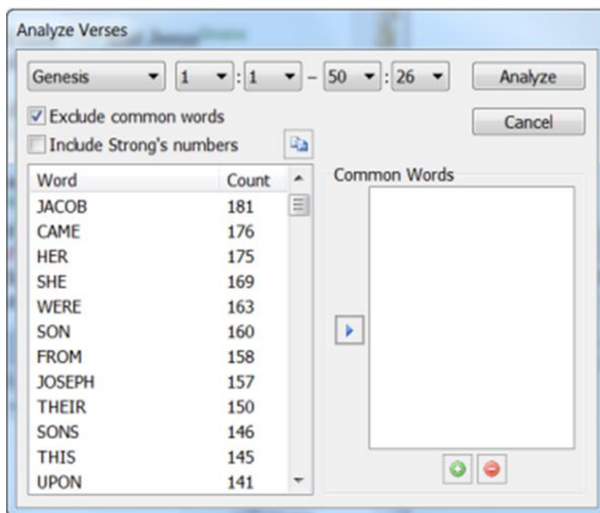
Εικόνα 49: Analyze Verses-e-Sword..
