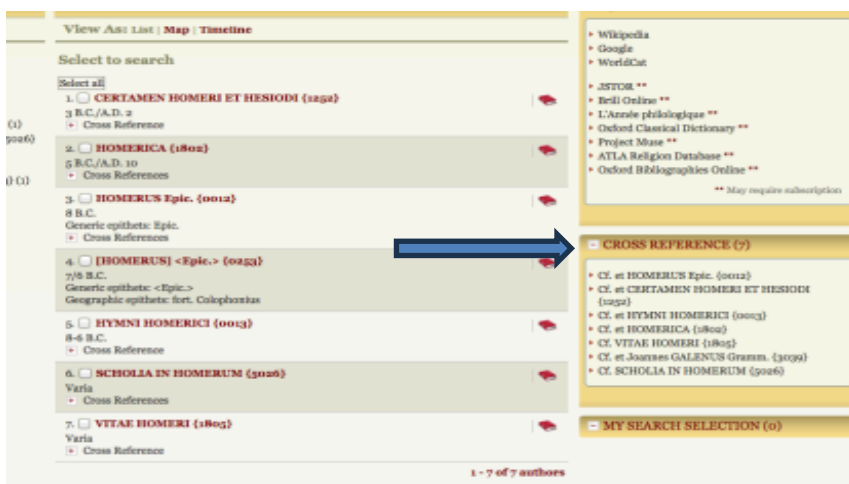
Εικόνα 9: CANON cross-references-TLG.
