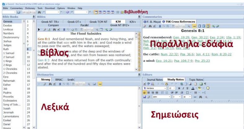
Εικόνα 41.: Διεπαφή e-Sword.
