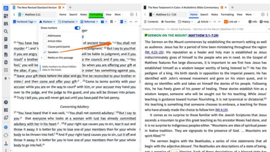
Εικόνα 63: Καρτέλα Formating-Logos.
