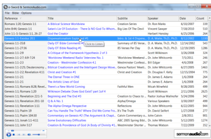
Εικόνα 52: SermonAudio.com - e-Sword.
