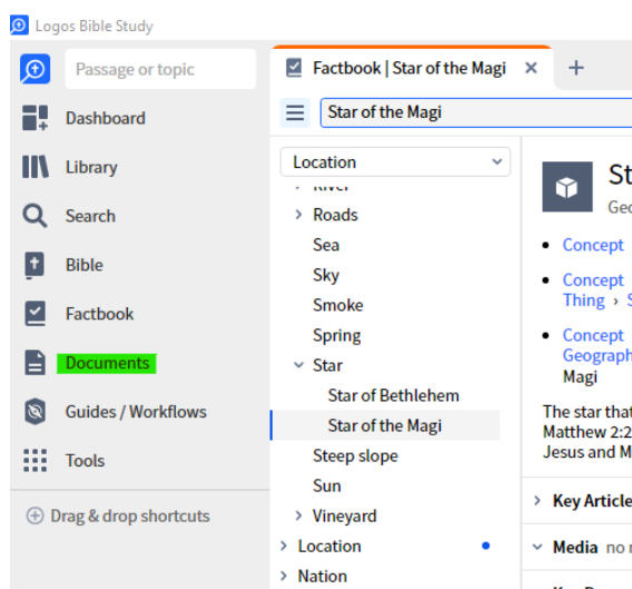
Εικόνα 61: Καρτέλα Έγγραφα-Logos
