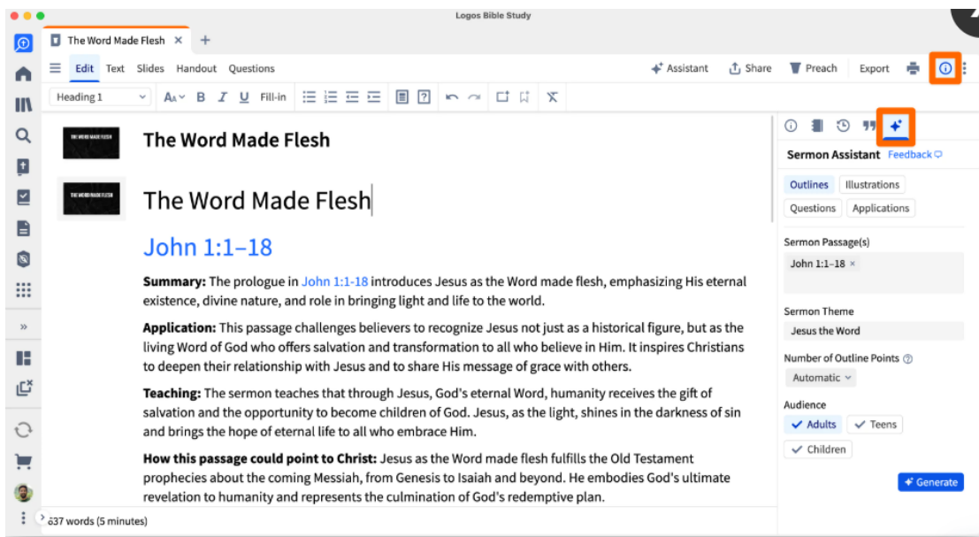
Εικόνα 72: Sermon Assistance-Logos.
