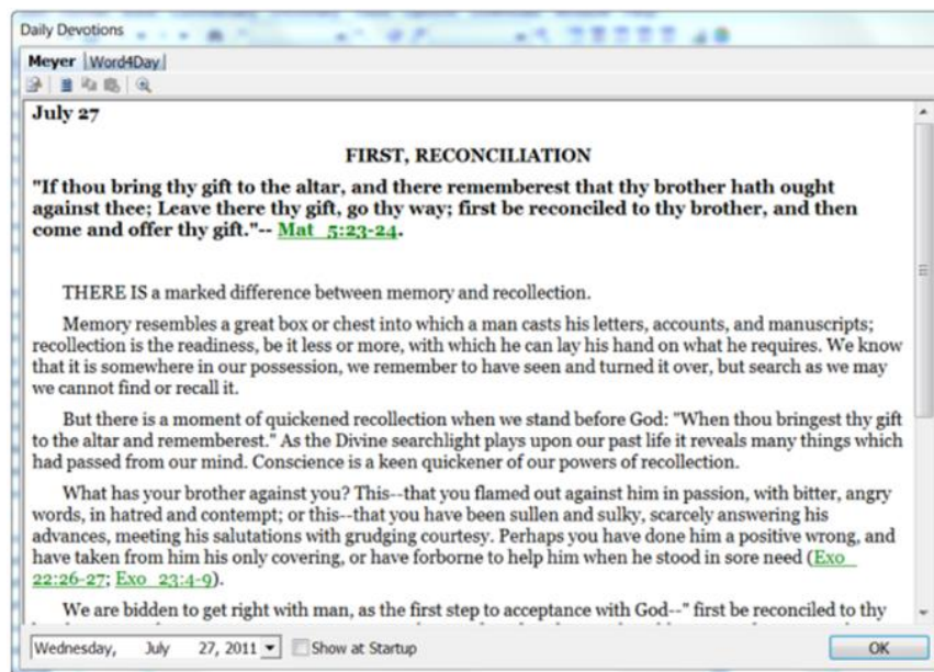
Εικόνα 44: Καθημερινά αναγνώσματα-e-Sword..
