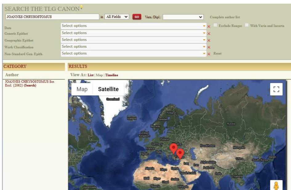
Εικόνα 5: Canon Map-TLG.
